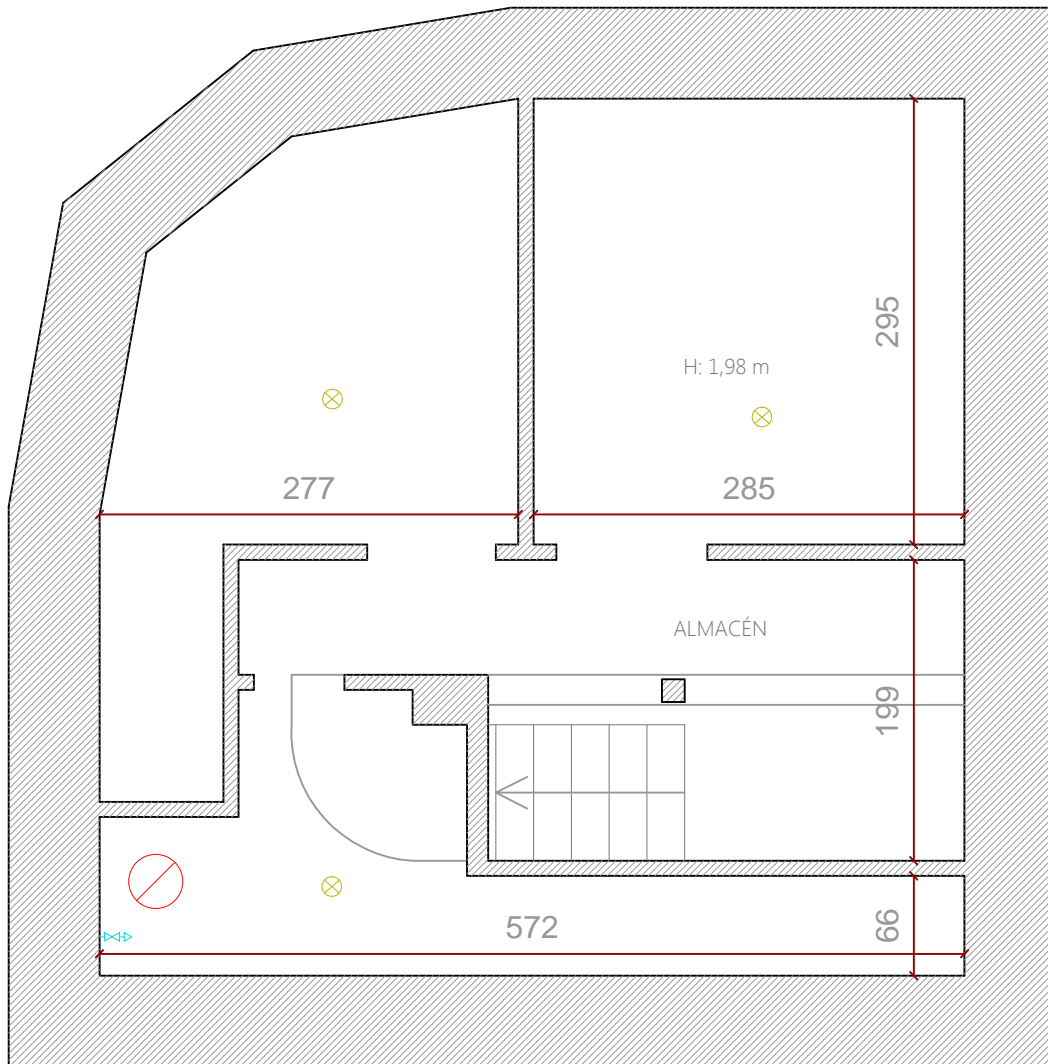
PLANTA SÓTANO (-1)
