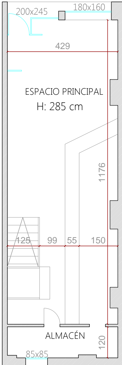
PLANTA BAJA
