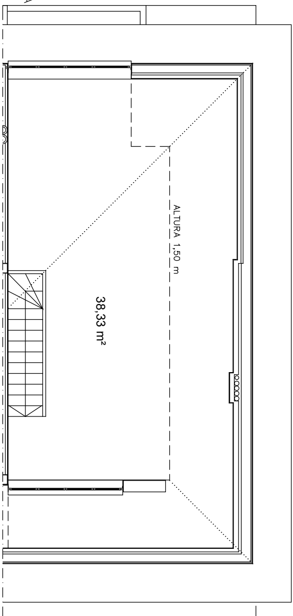
BAJO-CUBIERTA SUP útil 38,33 m 2
