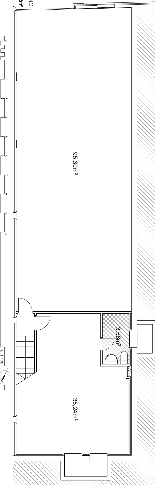
PLANTA SÓTANO SUP útil 134,12m 2
